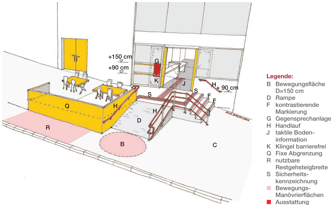
Bild 3: Stufe neben Rampe mit Handläufe und Markierungen
